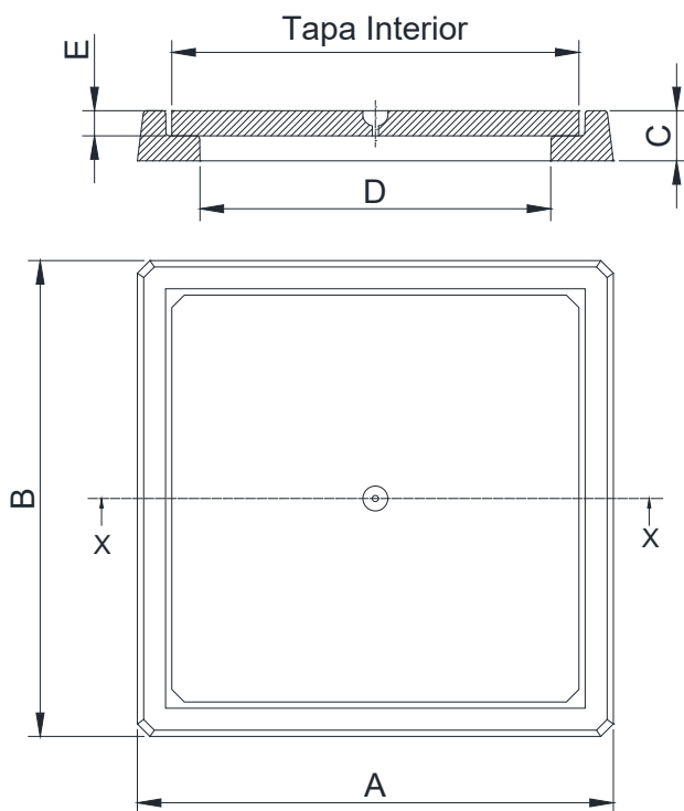
Sección XX:
